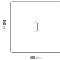
Fußplatte für klappbare Poller 8 mm dick
