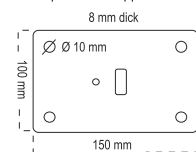
Fußplatte für klappbare Poller
