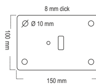
technische Daten der Fußplatten für klappbare Pfosten
