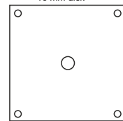
Fußplatten - Abmessung für Pfosten ab Ø 273 mm 360 x 360 mm 10 mm dick
