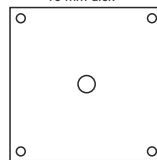
Fußplatten - Abmessung für Pfosten Ø 193 mm 300 x 300 mm 10 mm dick
