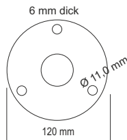
techn. Daten der Fußplatte für Pfosten Ø 48 mm und Ø 60 mm
