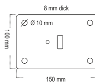
Abmessung der Fußplatte
