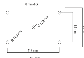
Fußplatten - Abmessung für Pfosten Ø 108 mm
